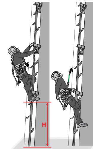
Şekil -3.1 Düşüş Öncesi Figure - 3.1 Before Fall
